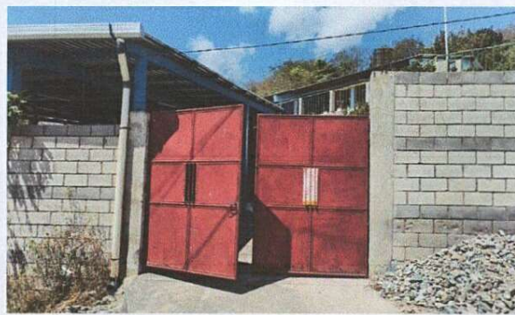
Foto 4: El portón tiene la deficiencia de no contar con una viga en la parte superior en donde se fijarían los pasadores, debido a ello se ha desprendido en varias ocasiones y se ha dañado la chapa de abertura.
